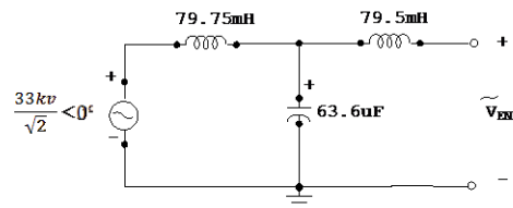
Fig. 2.1. Ferranti rise on no- load.
