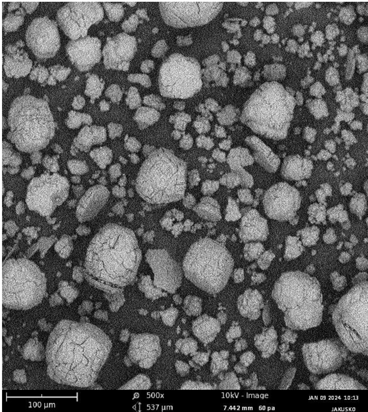
Figure 10: SEM Analysis (Jakusko)
